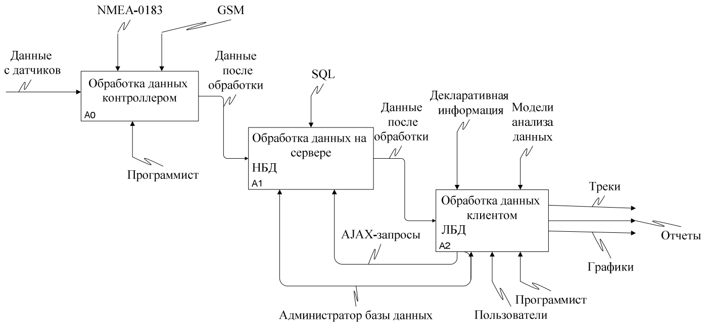
Рис. 1. Структура компьютерной технологии системы спутникового мониторинга
