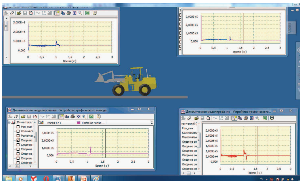
Рис. 10. Визначення опорних реакцій при різкому гальмуванні навантажувача Cat
