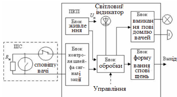
Рис. 3. Узагальнена функціональна схема приймально-контрольного приладу малої інформаційної ємкості
